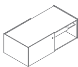
V36M 1602 / 784 / 545 96.5 kg
