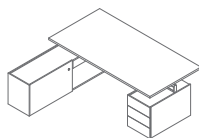
V10LM 2000 / 1800 / 740 203.22 kg
