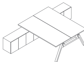
V2024 2000 / 3200 / 740 287.2 kg
