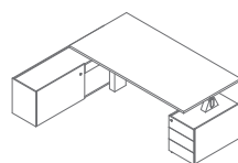
V10LR 2000 / 1000 / 740 210.22 kg
