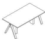
V01R 1800 / 1000 / 740 99.66 kg
