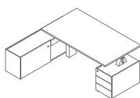
V09LR 1800 / 1000 / 740 202.16 kg
