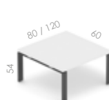
MWSK 0860 U 80 / 60 / 54 [22]
