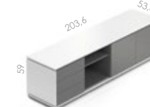
MWKB 3011 203,6 / 53,6 / 59 [174]
