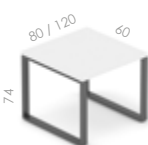
MWSK 0860 WO 80 / 60 / 74 [28]
