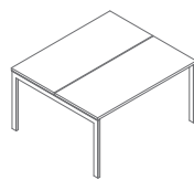
BOU54 1400 / 1210 / 740 54 kg
