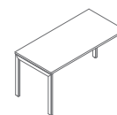
BOU30 1600 / 700 / 740 61.55 kg
