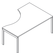
BOU25 1800 / 1200 / 740 51.2 kg
