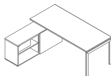
BOUL21 1800-1902 / 1600 / 740 107.15 kg
