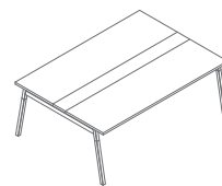
SW48 1800 / 1410 / 740 72 kg
