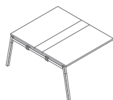
SW42L 1200 / 1410 / 740 45.2 kg
