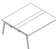
SW34L 1600 / 1610 / 740 65 kg
