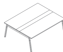
SW35 1800 / 1610 / 740 79 kg
