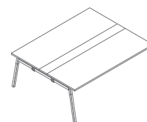
SW35L 1800 / 1610 / 740 72.8 kg
