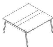
SW44 1400 / 1410 / 740 57 kg
