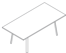
PLF12PK 2000 / 800-1000 / 740 45 kg
