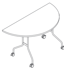
PFT06 695 / 1390 / 740 26.3 kg
